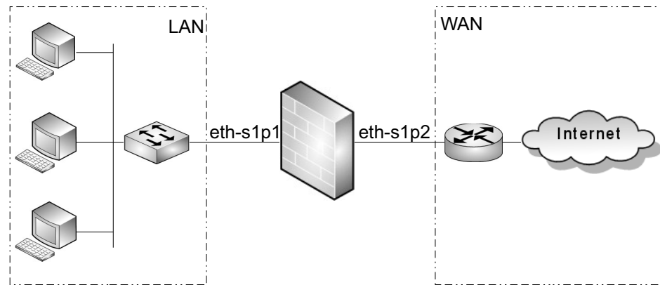
图 15 UTM 客户端防护典型应用
