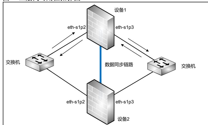
图 2 三层高可用性拓扑图
