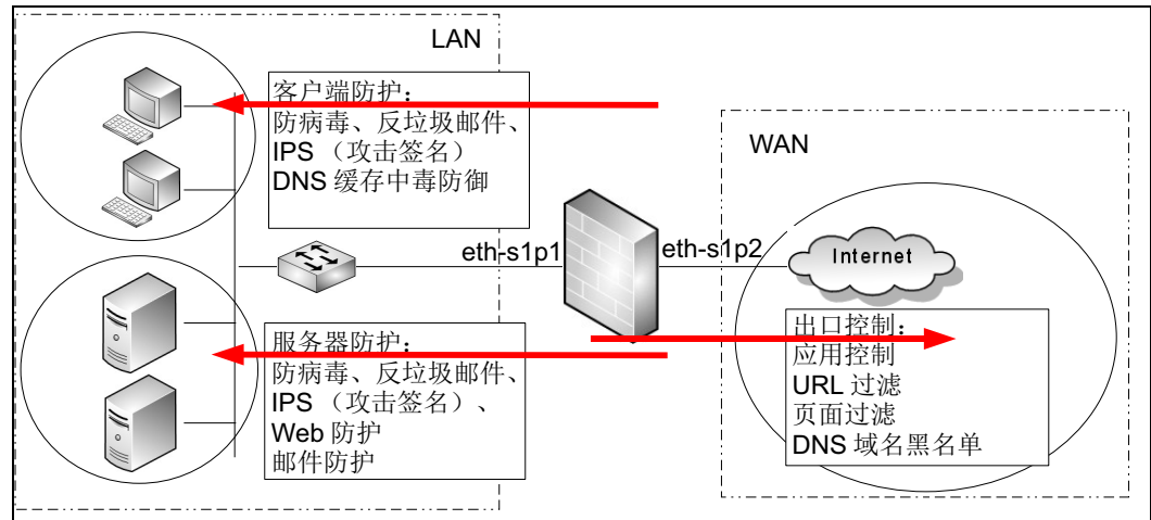
图 13 UTM 典型应用场景
