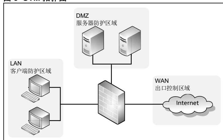
图 5 UTM 拓扑图
