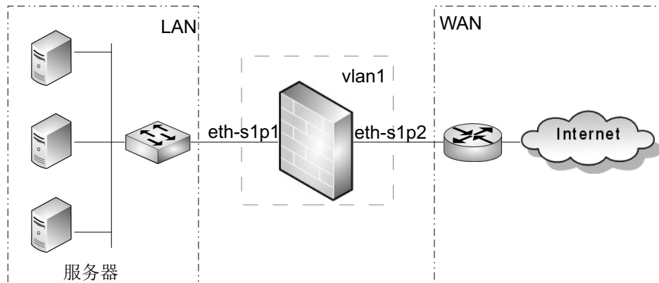
图 16 UTM 服务器防护典型应用
