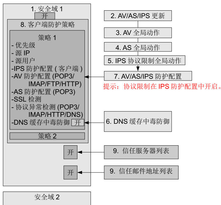
图 18 客户端防护配置步骤
