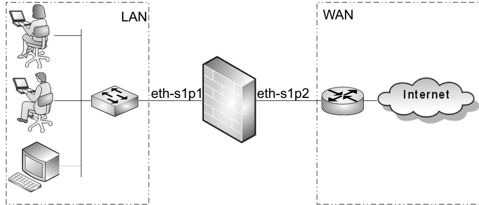
图 14 UTM 出口控制典型应用
