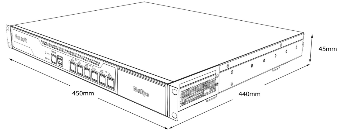
图 1 整机示意图
