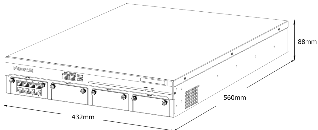
图 1 整机示意图
